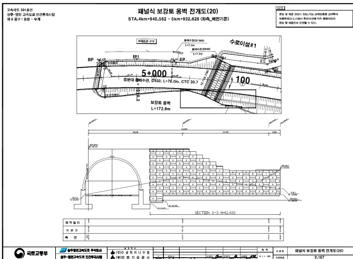
【그림 73.4】 전개도
