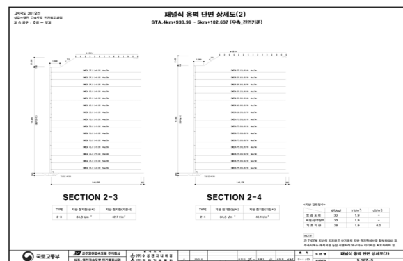
단면도
