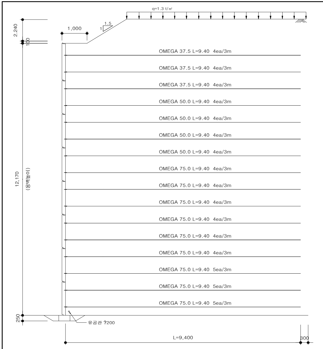
【그림 73.10】 검토단면도
