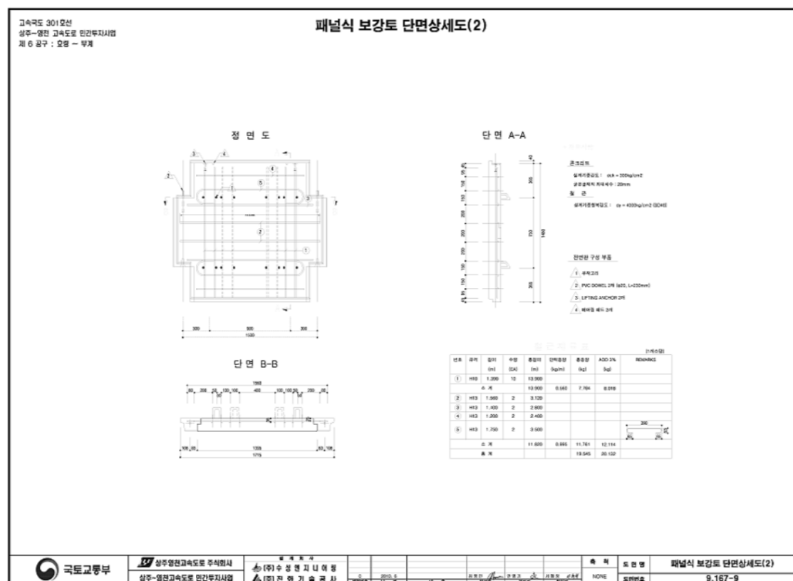
【그림 7.5】 단면도(계속)
