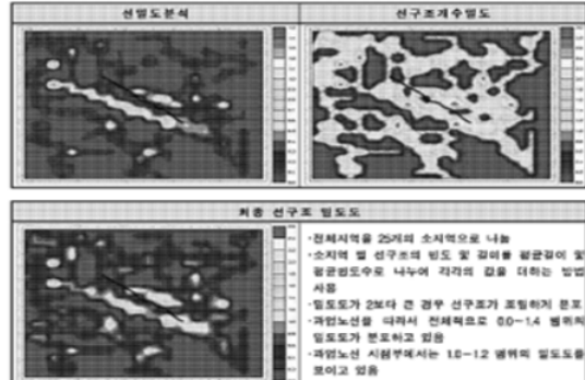
대. 선구조 밀도분석
